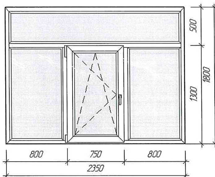
Схема планирцемых к установке окон ПВХ
